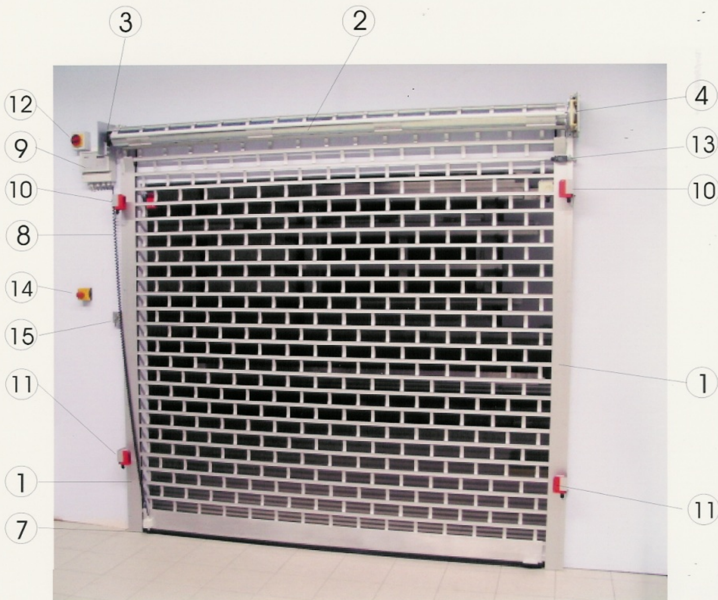
Rollgitter Typ A3601 + B3602
